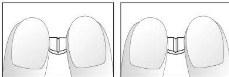
Pictogramele 3 și 4: Ruperea ușoară în sferturi a unei jumătăți de comprimat de Nolet 5 mg
